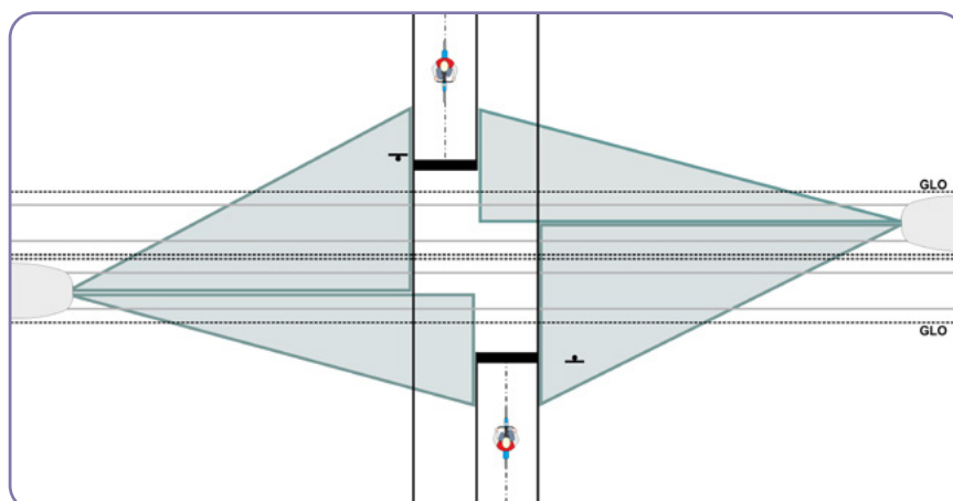
Schéma 1 : pour une même traversée, la visibilité doit être dégagée pour chaque sens de circulation du tiers et du tramway.
