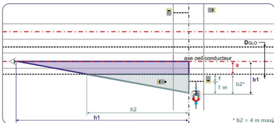
Schéma 13 : cône de visibilité pour une traversée cyclable gérée par signalisation lumineuse.
