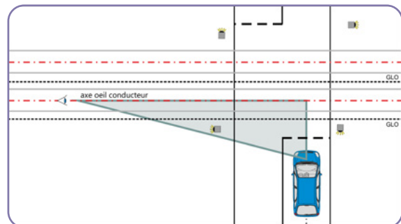
Schéma 3 : exemple de dégagement de la visibilité pour une traversée automobile gérée par signalisation lumineuse.
