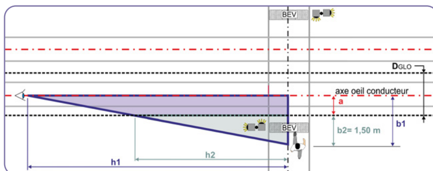
Schéma 11 : cône de visibilité pour une traversée de voies tramways aménagée pour les piétons gérée par signalisation lumineuse.
