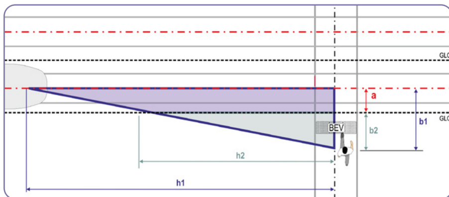
Schéma 5 : construction de la zone libre de masque (triangle h2, b2) à partir du cône de visibilité (h1, b1).
