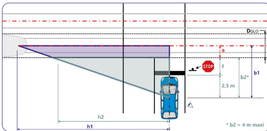
Schéma 9 : cône de visibilité pour une traversée automobile avec signalisation statique.
