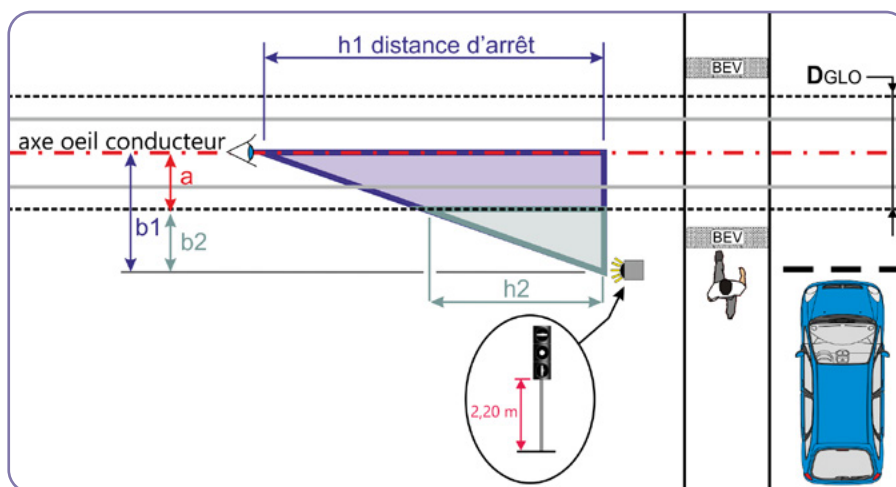
Schéma 15 : cône de visibilité pour la visibilité sur les signaux destinés au conducteur tramway.
