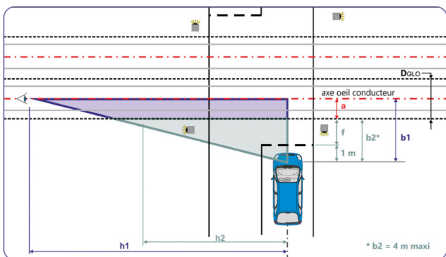
Schéma 14 : cône de visibilité pour une traversée automobile gérée par signalisation lumineuse.
