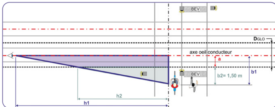
Schéma 12 : cône de visibilité pour une traversée cycle contiguë à une traversée de voies tramways aménagée pour les piétons gérée par signalisation lumineuse.
