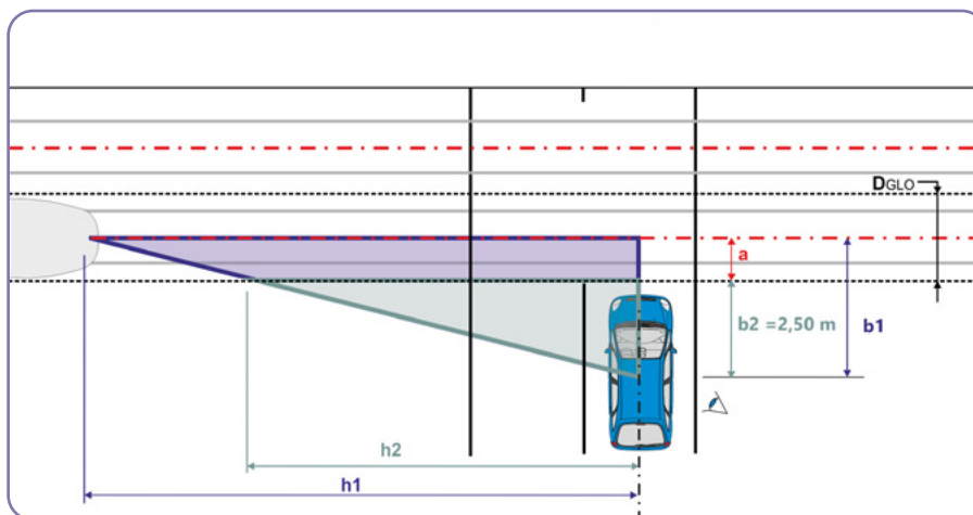
Schéma 10 : cône de visibilité pour une traversée automobile avec absence de marquage au sol.
